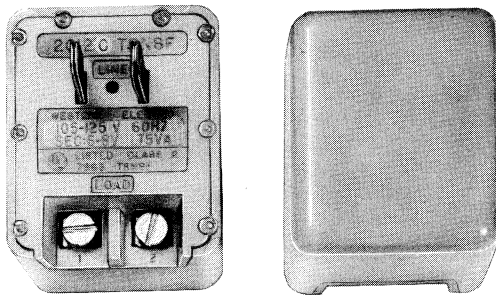
Fig. 6—2012C Transformer
