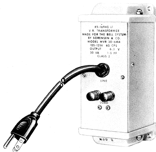
Fig. 9—KS-16940L1 V.R. Transformer
